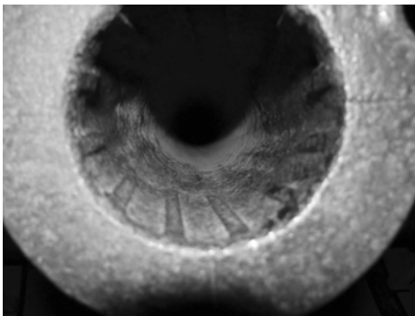
De eerste getrokken loop van Thyssen
